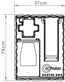
Cotes extérieures
