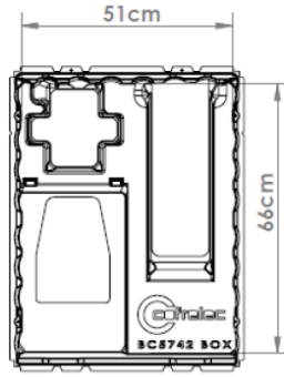
Cotes intérieures
