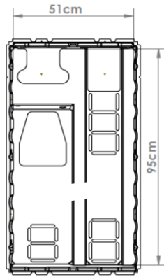
Cotes intérieures
