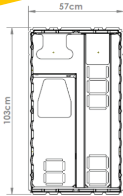
Cotes extérieures
