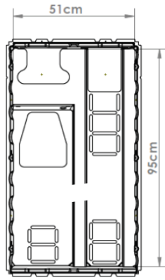
Cotes intérieures
