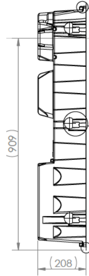
Coupe C-C
