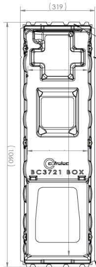
Cotes extérieures
