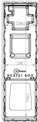
Cotes intérieures
