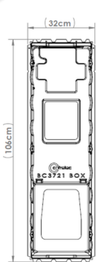
Cotes extérieures
