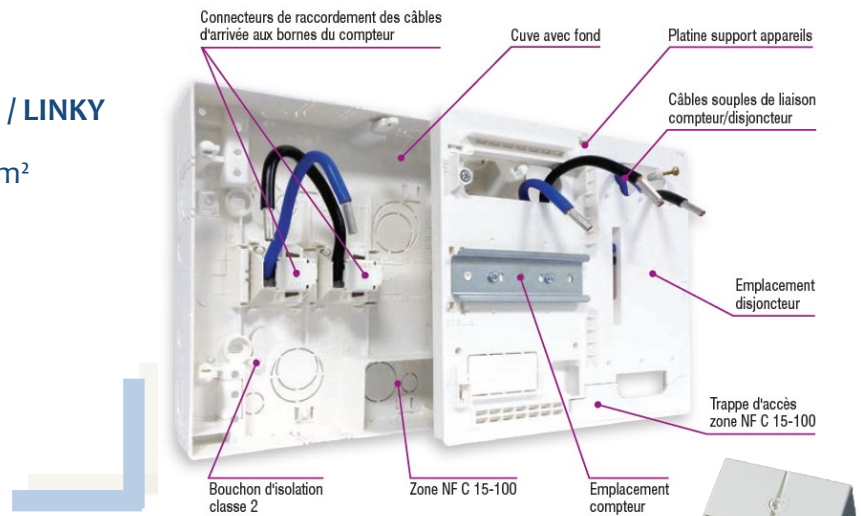
Platine + disjoncteur
